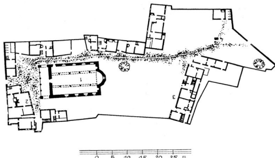
обр. 9. План на метоха и Храм „Покров Пресвятия Богородици“ (1837– 839 г.), в гр. Самоков, архитектурно заснемане от Тодор Златев (Коева 2002: 248)
